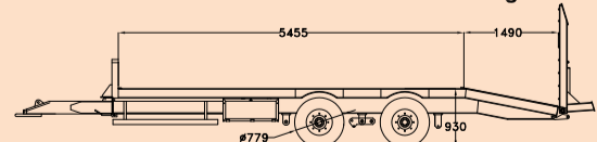
PE 150 TANDEM PTAC : 19 000 kg CU : 15 000 kg
