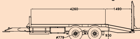
PE 90 PTAC : 12 000 kg CU : 9 200 kg
