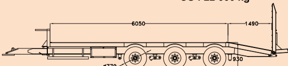
PE 220 TRIDEM PTAC : 27 000 kg CU : 22 000 kg
