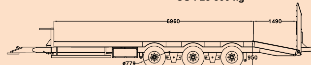
PE 320 TRIDEM PTAC : 32 000 kg CU : 25 500 kg
