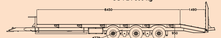
PE 320 TRIDEM L PTAC : 32 000 kg CU : 24 500 kg
