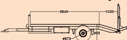
PE 60 PTAC : 8 000 kg CU : 6 000 kg
