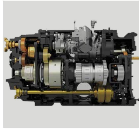
Transmission CVX – une conduite en continu de 0 à 40 km/h.
